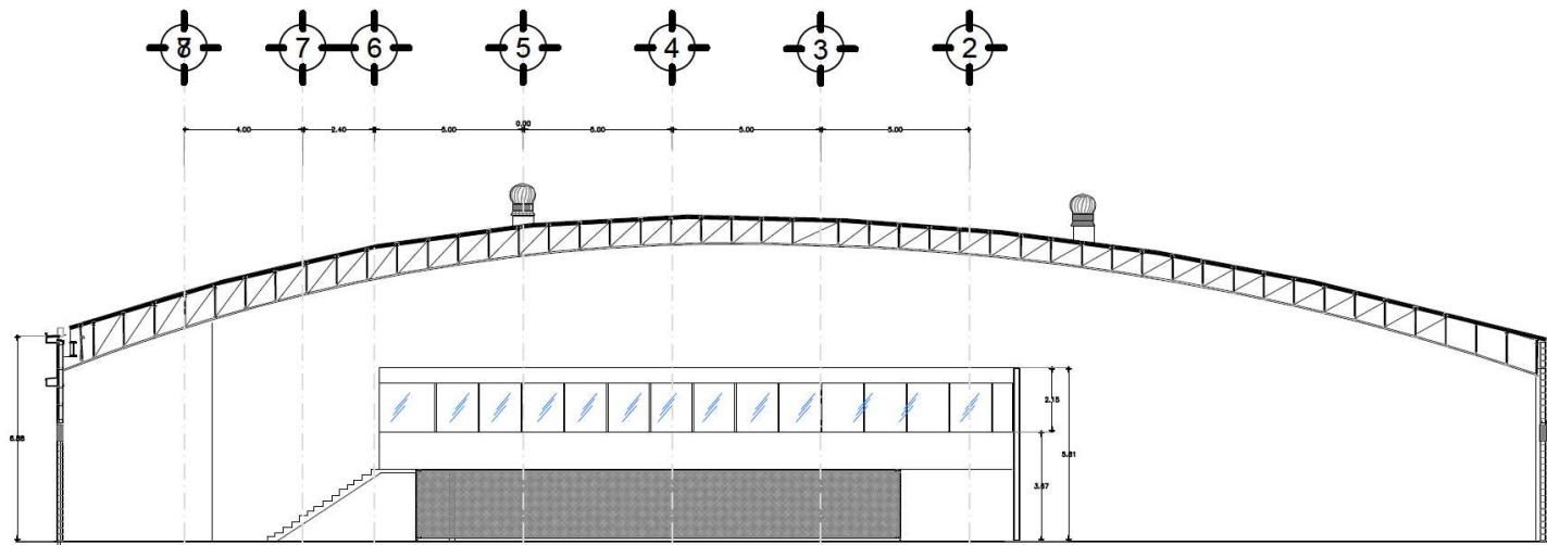
ALZADO
